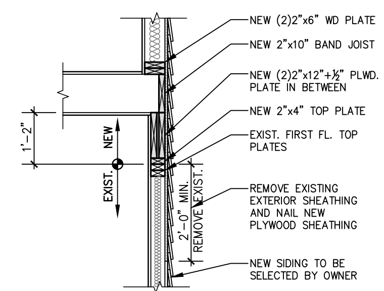
DETAIL 1 SCALE: 1/2"=1'-0"
